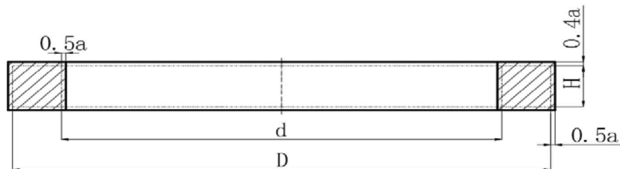
图2 环形锻件轮廓图
