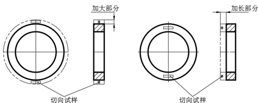
图3 环形锻件取样位置
