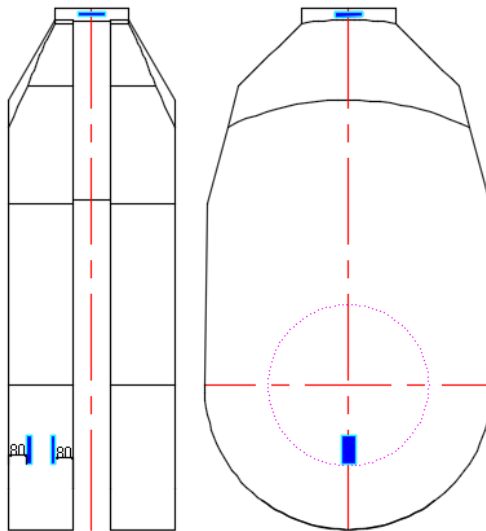
图1 模锻曲拐锻件取样要求
